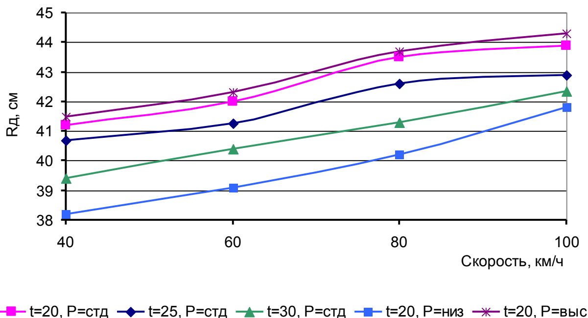
Рис. 3. Зависимость динамического радиуса от скорости движения при различных значениях температуры и давления в шине
