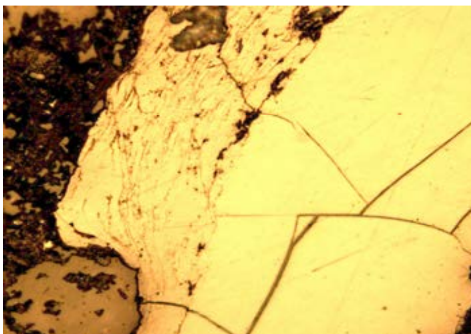
Рис. 1. Обр. 2961. Структурный витринит – телинит с сохранившимся клеточным строением (слева) и однородный бесструктурный витринит – коллинит (справа). Ув. 200 х
