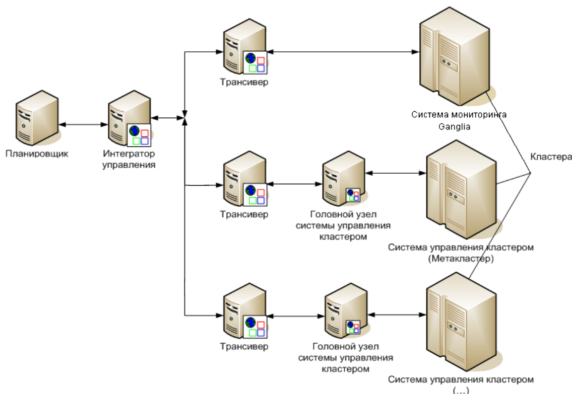
Рис. 1. Архитектура программного компонента управления платформами исполнения MCMS
