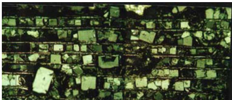
Рис. 1. Микрофотография текстурированной ВТСП-керамики
