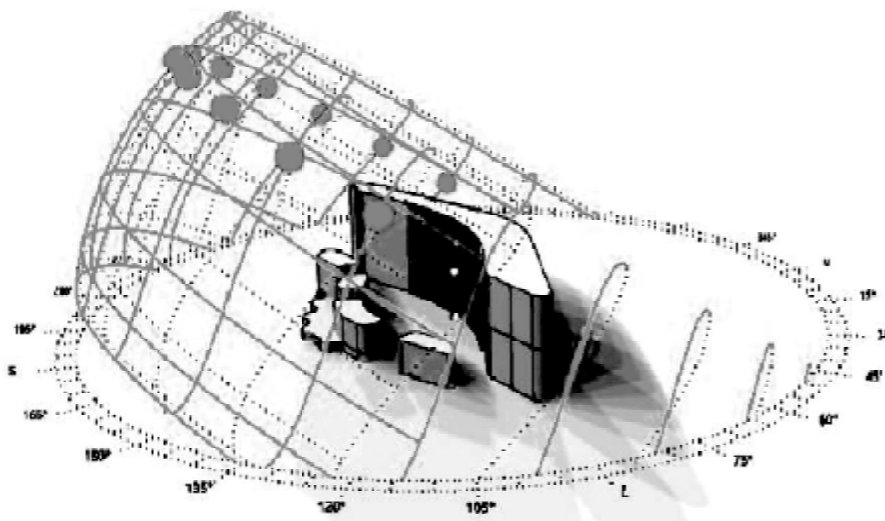
Рис. 5. Расчетная модель основного и отражающего здания. Разбиение сетки для учета отраженных лучей (иллюстрация авторов)
