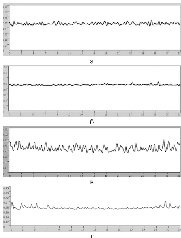
Рис. 3 – Рельеф поверхности стали 9ХФ до ВЧ плазменной обработки (а) и после (б), и стали У8 до ВЧ плазменной обработки (в) и после (г)
