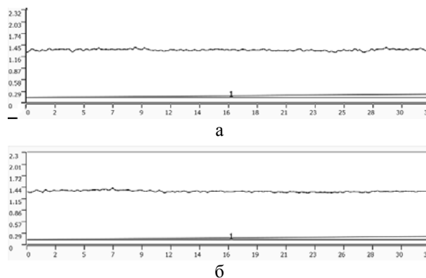
Рис. 1 – Рельеф поверхности стали 9ХФ до обработки в тлеющем разряде (а) и после (б)
