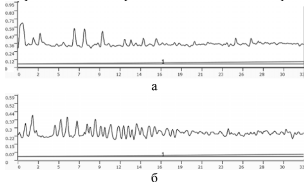
Рис. 2 – Рельеф поверхности стали У8 до обработки в тлеющем разряде (а) и после (б).
