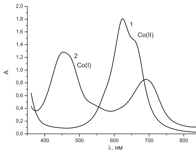
Рисунок 1. Исходный (1) и конечный (2) спектры, полученные при исследовании восстановления \text{Co}^{\text{II}}(\text{TSPc})^4 глюкозой; [глюкоза] = 0.1 моль/л, [\text{Co}^{\text{II}}(\text{TSPc})^4] = 3.0 \cdot 10^{-5} моль/л, 0.1 моль/л NaOH, 298 K.
