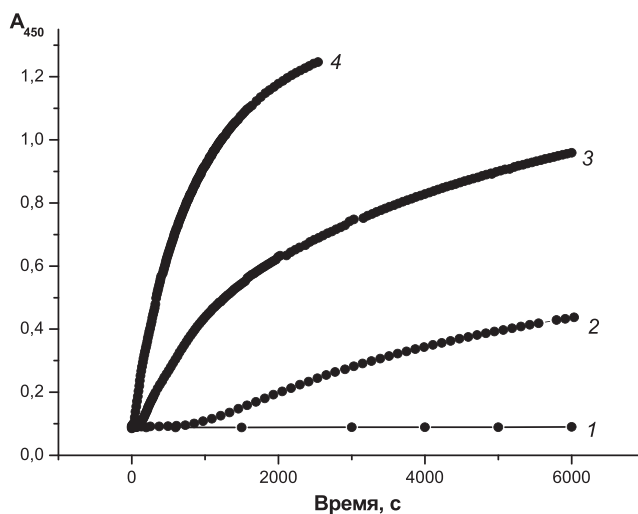
Рисунок 2. Изменение оптической плотности при 450 нм в процессе восстановления \text{Co}^{\text{II}}(\text{TSPc})^4 глюкозой при pH 10.0 (1), 11.6 (2), 12.3 (3), 12.8 (4), [глюкоза] = 0.1 моль/л, [\text{Co}^{\text{II}}(\text{TSPc})^4] = 3.0 \cdot 10^{-5} моль/л, 298 K.
