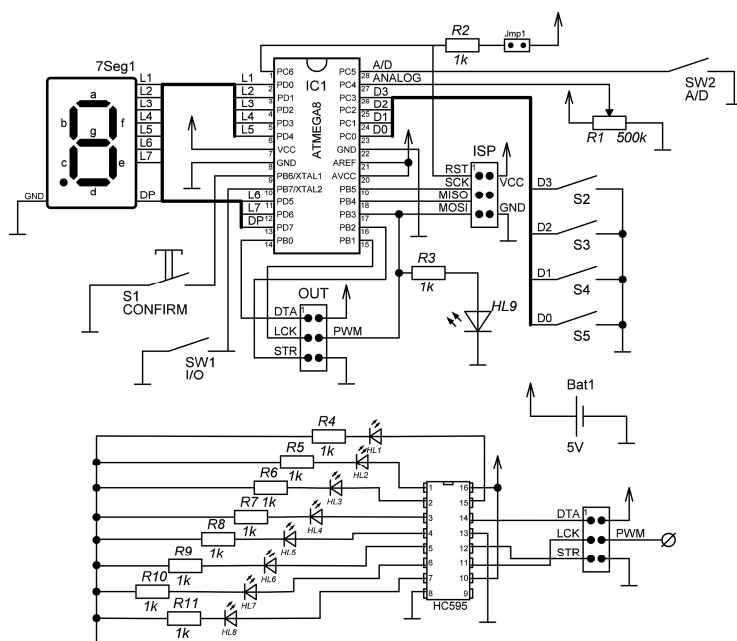
Рис. 1. Принципиальная схема устройства
