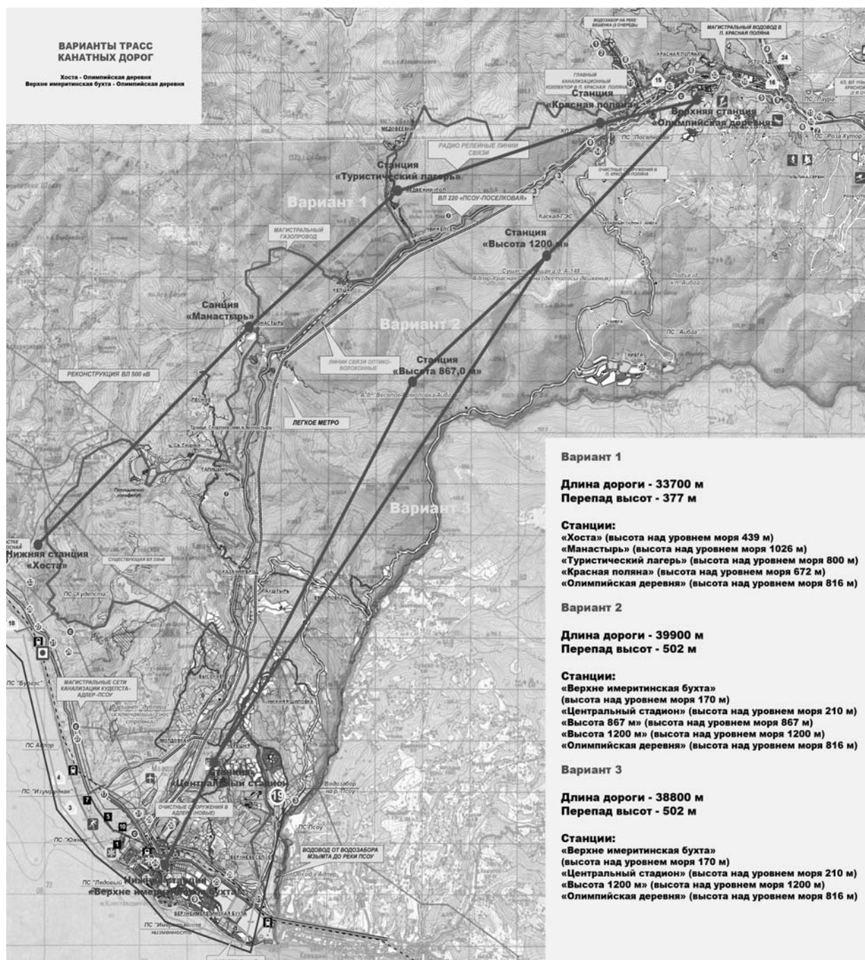
Рис 1. Три варианта трассы канатной дороги
