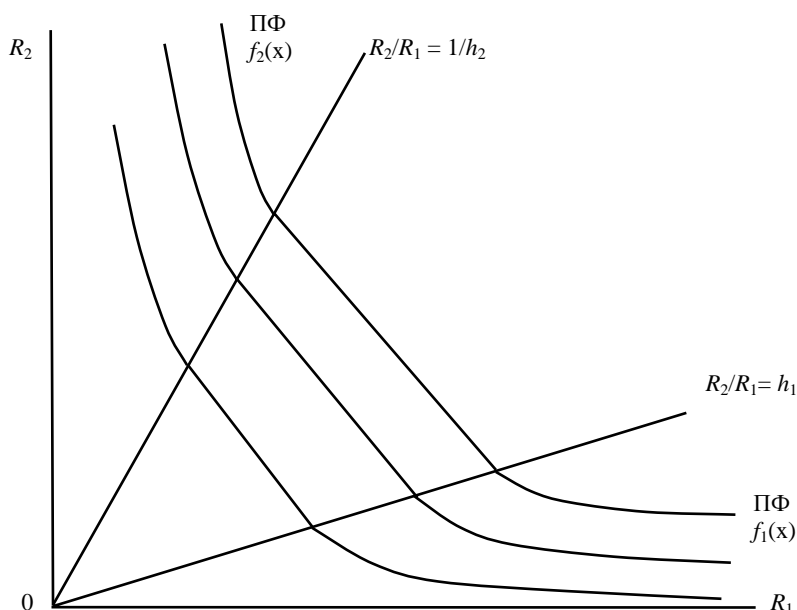
Рис. 3. Линии уровня КПФ (режим композиции существует) F(R_1, R_2) = \max_{X \in \Omega(R)} \{A_1 x_{11}^{a(1,1)} x_{12}^{1-a(1,1)} + A_2 x_{21}^{1-a(2,2)} x_{22}^{a(2,2)}\}
