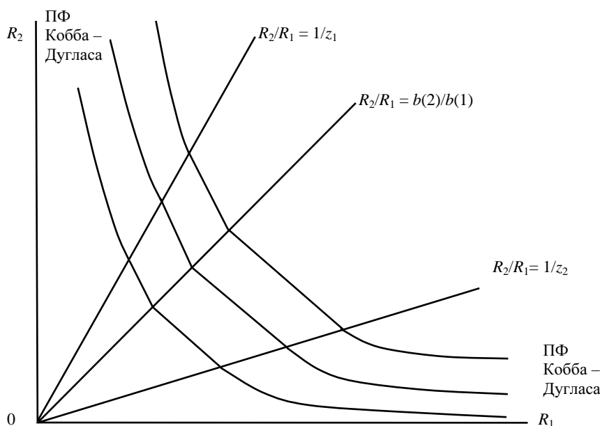
Рис. 2. Линии уровня КПФ (режим композиции существует)
