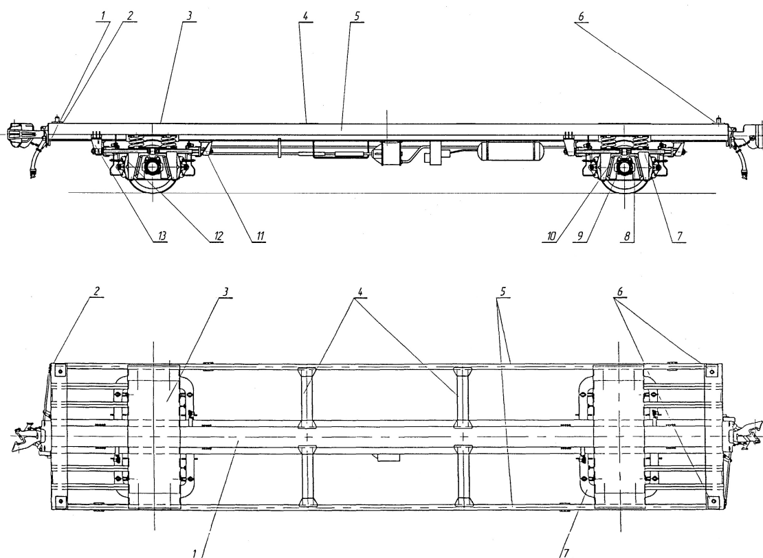
Рис. Специализированная двухосная платформа для перевозки контейнера: 1 – хребтовая балка рамы; 2 – лобовая балка рамы; 3 – наддрессорная балка рамы; 4 – промежуточная поперечная балка рамы; 5 – продольная обвязка рамы; 6 – фитинговый упор; 7 – рама тележки; 8 – кузовная ступень подвешивания тележки; 9 – букса; 10 – надбуксовая ступень подвешивания тележки; 11 – ограничительный упор; 12 – продольный тяговый поводок; 13 – кронштейн
