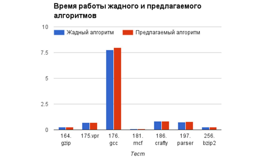
Диаграмма 6. Сравнение времени работы разработанного алгоритма с жадным Diagram 6. Run time comparison of proposed algorithm vs greedy
