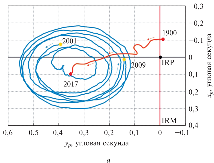
Рис. 3 (начало). Траектория движения полюса ( 0,1 угловой секунды \approx 3 м в проекции на поверхность Земли):
