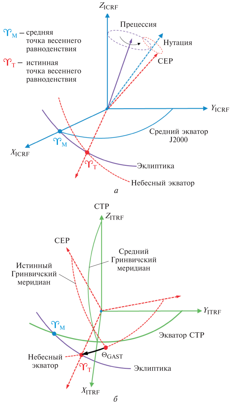
Рис. 1. Определение систем координат:
