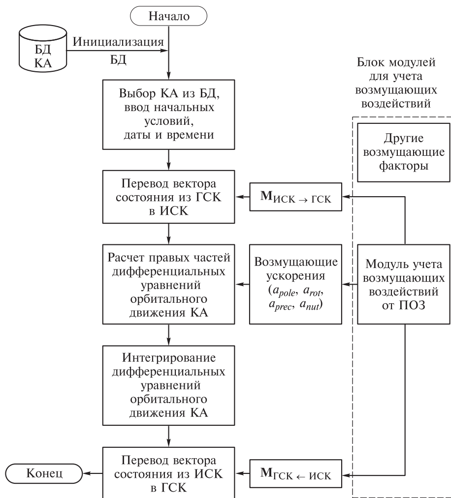
Рис. 5. Блок-схема работы ПАК
