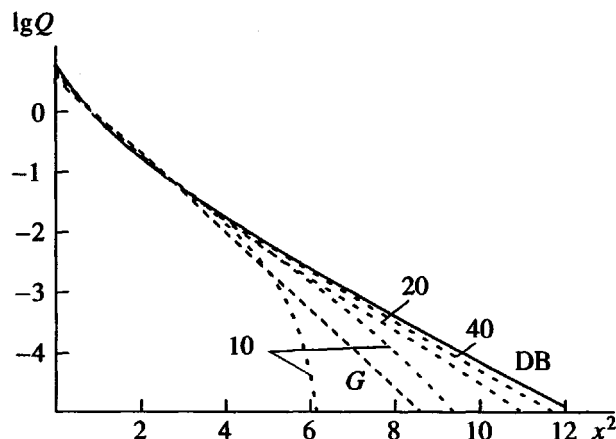
Рис. 2. Графики логарифмов безразмерных распределений плотности, рассчитанные на основании модели свободносочлененных сегментов (штриховые линии, цифры у которых показывают число сегментов), и для распределения Деbye–Бюеche (сплошная кривая DB). Прямая G соответствует гауссовому распределению плотности.
