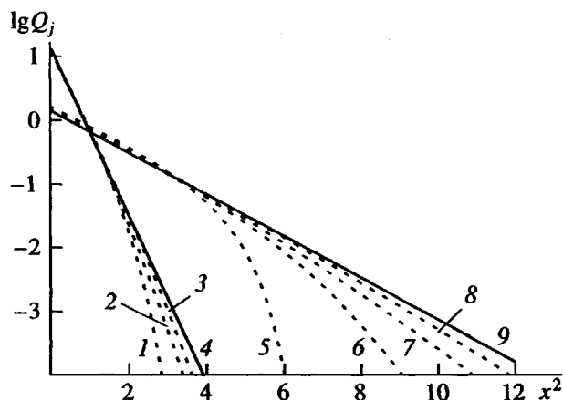
Рис. 1. Графики логарифмов безразмерных распределений расстояний центральной (1–4) и концевой (5–9) бусин от центра масс клубка, рассчитанные согласно модели свободносочлененных сегментов с N = 10 (1, 6), 20 (2, 7), 40 (3, 8) и 5 (5), в сравнении с прямыми (4, 9), соответствующими гауссовым распределениям (7).
