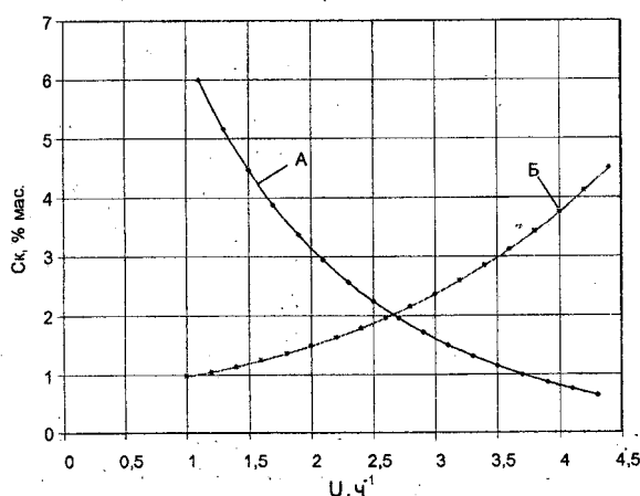
Рис. 3. Распределение концентрации кокса на катализаторе
