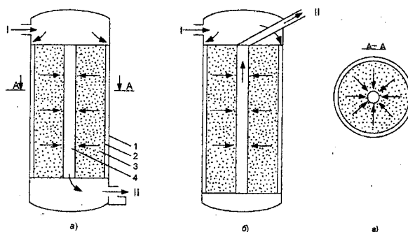
Рис. 1. Схема движения газового потока в радиальном реакторе: корпус аппарата, 2) катализаторная корзина, 3) катализатор, 4) коллектор: 1 – гидрогенизатор, II – катализатор
