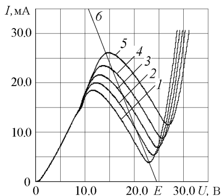
Рис. 3. Рассчитанные ВАХ нелинейного двухполусника при различных значениях внешнего магнитного поля B : 1 – (–180) мТл; 2 – (–90) мТл; 3 – 0; 4 – 90 мТл; 5 – 180 мТл; 6 – нагрузочная прямая
