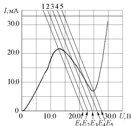
Рис. 4. Рассчитанная ВАХ нелинейного двухполусника при фиксированном значении B = 0 и семейство нагрузочных прямых 1–5, имитирующих изменение величины внешнего магнитного поля
