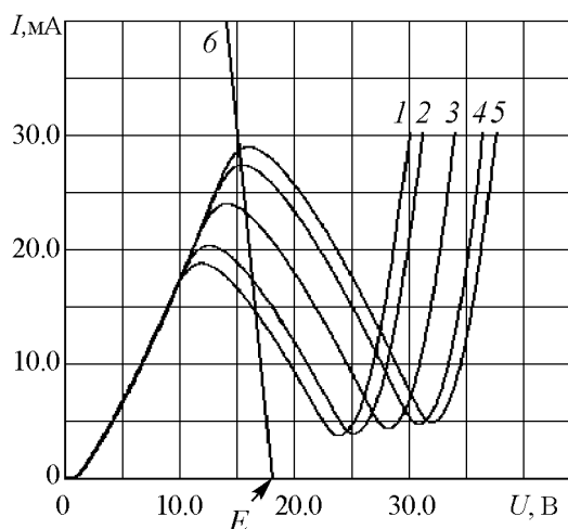
Рис. 11. Рассчитанные ВАХ нелинейного двухполосника при различных значениях температуры T : 1 – 27^\circ\text{C} ; 2 – 35^\circ\text{C} ; 3 – 55^\circ\text{C} ; 4 – 75^\circ\text{C} ; 5 – 85^\circ\text{C} ; 6 – нагрузочная прямая
