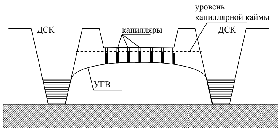
Рисунок – Физическая модель испарения с поверхности понижающихся грунтовых вод
