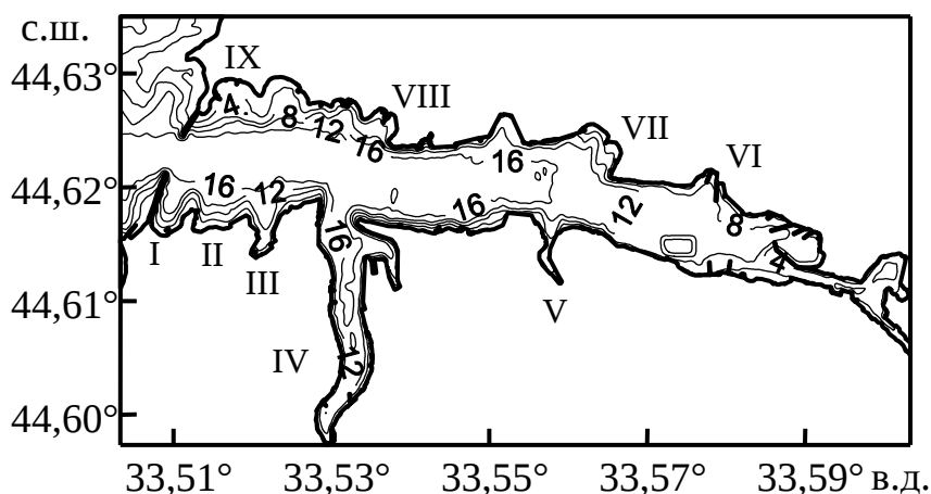
Рис. 1. Батиметрия Севастопольской бухты (м). Римскими цифрами обозначены: I – Мартинова бухта; II – Александровская бухта; III – Артиллерийская бухта; IV – Южная бухта; V – Килен-бухта; VI – Сухарная бухта; VII – бухта Голландия; VIII – Северная бухта; IX – Константиновская бухта
