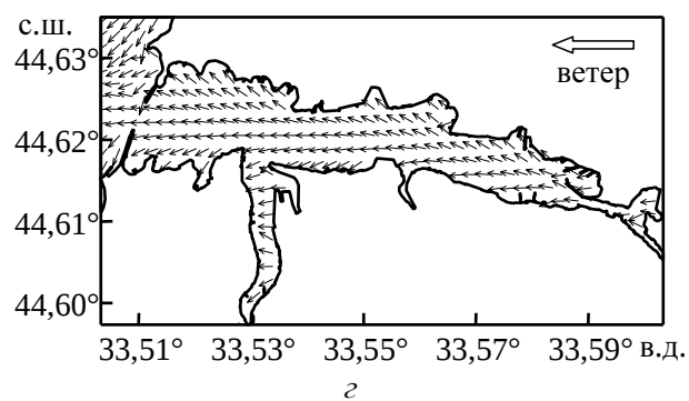
Р и с. 3. Направление распространения ветровых волн при разных направлениях ветра скоростью 20 м/с: a – при западном ветре; б – при южном; в – при северном; г – при восточном
