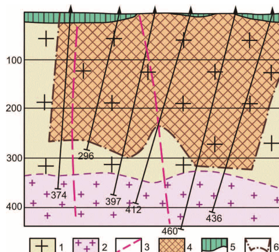
Рис. 5. Геологический разрез по одному из разведочных профилей месторождения Каскырказган (составил С.А. Акылбеков). 1 – лейкократовые гранит-порфиры (C 2-3 ); 2 – граниты средне-крупнозернистые (D 3 ); 3 – тектонические нарушения (а), поисково-разведочные скважины; 4–5 – медно-молибденовые руды: 4 – сульфидные, 5 – окисленные; 6 – контур подсчета запасов
