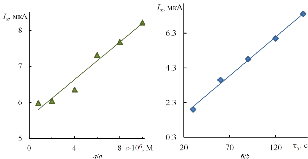
Рис. 6. Зависимости величины максимума катодного тока ртутно-пленочного электрода (а) от концентрации \text{Na}_2\text{S}_2 (фон 0,1 М NaOH) без предэлектролиза и (б) от продолжительности предэлектролиза \tau_3 при E_3 = -0,5 В в растворе 4 \cdot 10^{-7} М \text{Na}_2\text{S}_2 + 0,1 М NaOH по данным переменноточковой вольтамперометрии ( E_{\text{нач}} = -0,5 В; E_{\text{кон}} = -1,1 В; v = 40 мВ/с; \Delta U = 3 мВ; \theta = 0^\circ ; f = 25 Гц)
