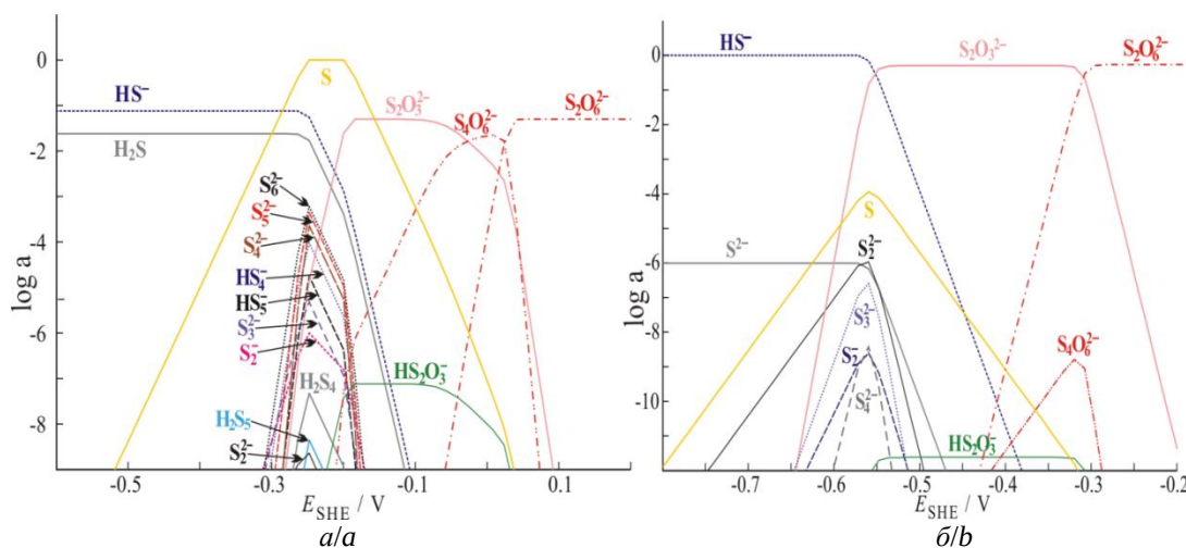
Рис. 2. Расчетные зависимости логарифмов равновесных активностей ионно-молекулярных форм от потенциала (с. в. э.) в системе S–H 2 O (без учета SO 4 2- ) при pH 7,5 (а) и 13 (б) (25 °C; [S] общ =0,1 М)
