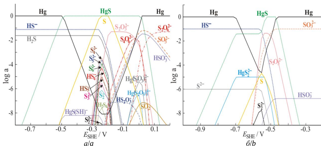
Рис. 3. Расчетные зависимости логарифмов равновесных активностей ионно-молекулярных форм от потенциала (с. в. э.) в системе Hg–S–H 2 O (без учета SO 4 2- ) при pH 7,5 (а) и 13 (б) (25 °C; [Hg] общ =1·10 -5 М; [S] общ =0,1 М)
