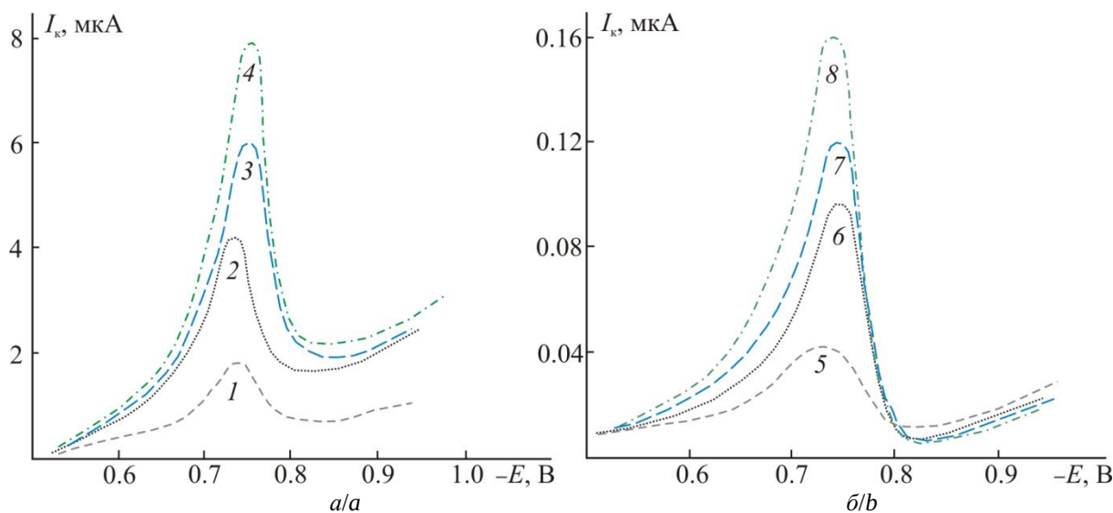
Рис. 7. Вольтамперограммы ртутно-пленочного электрода в растворах \text{Na}_2\text{S}_3 + 0,1 М NaOH в условиях линейной постоянноточковой (а) и переменноточковой (б) вольтамперометрии при различных концентрациях \text{Na}_2\text{S}_3 : 1) 4 \cdot 10^{-7} , 2) 6 \cdot 10^{-7} , 3) 8 \cdot 10^{-7} , 4) 1 \cdot 10^{-6} , 5) 2 \cdot 10^{-7} , 6) 6 \cdot 10^{-7} , 7) 8 \cdot 10^{-7} , 8) 1 \cdot 10^{-6} М ( E_{\text{нач}} = -0,5 В; E_{\text{кон}} = -1,1 В; v = 40 мВ/с; \Delta U = 3 мВ; \theta = 0^\circ ; f = 25 Гц)
