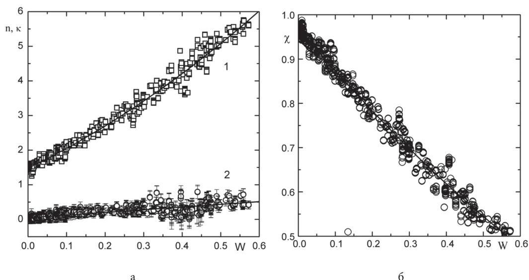
Рис. 2. Зависимости показателей преломления n (1) и поглощения k (2) от влажности для всех почв, отобранных с тестовых участков в бассейне Верхней Оби (а).
