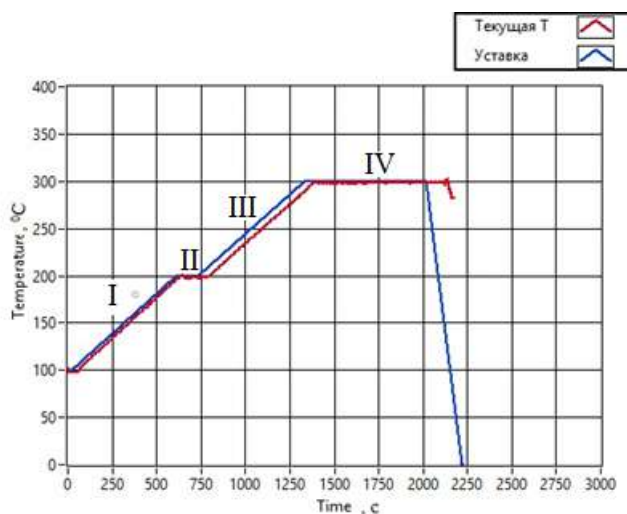
Рис. 2. Задаваемая (синяя кривая) и регистрируемая экспериментально (красная кривая) зависимости температуры испарителя от времени
