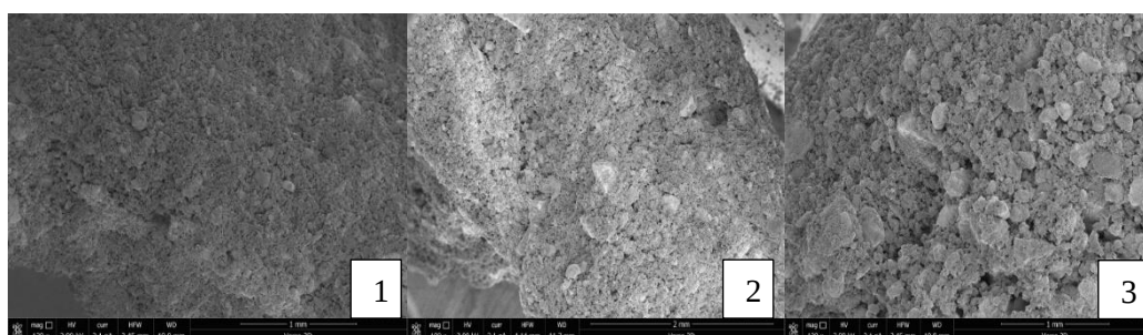
Рисунок 2. Структура поверхности состава: 1 – БГМКД-3; 2 – БГМКД-1; 3 – БГМКД-2; (сделано Агеевой А.С., описание составлено авторами)
