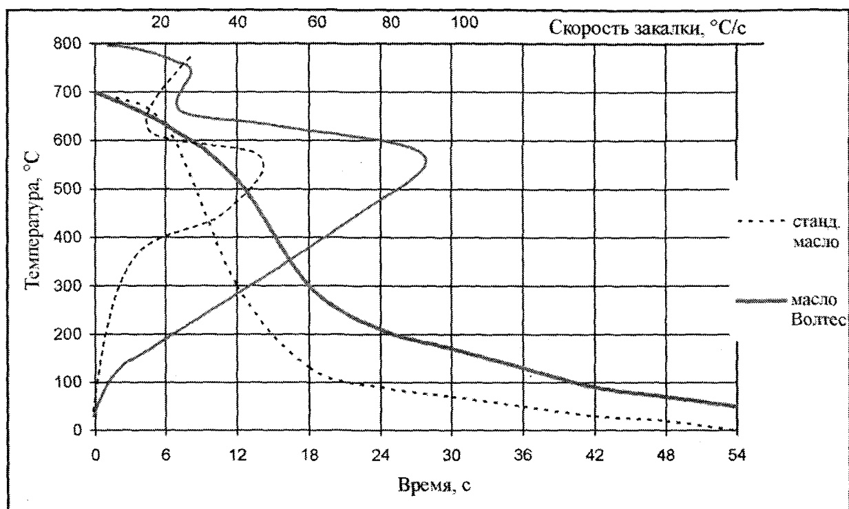
Сравнение закалочной способности стандартного индустриального масла и масла ВОЛТЕС МЗ (одинаковой вязкости в одинаковых условиях)
