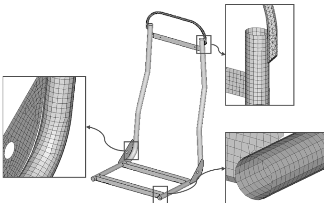
Рис. 2. Конечно-элементная модель
