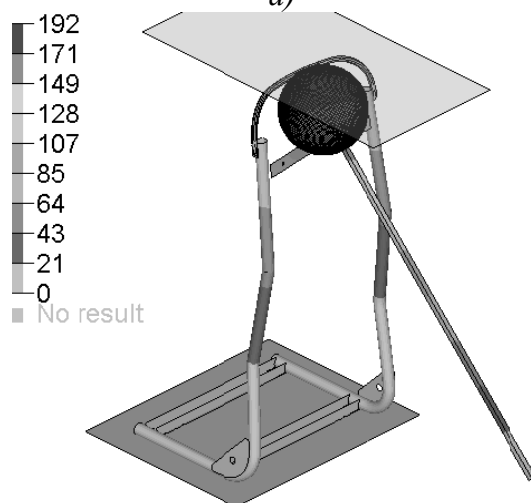
Рис. 4. Деформации каркаса сиденья
