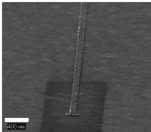
Рис.4. РЭМ фотография вытравленного рельефа активной области после снятия резистивной маски ( RF=125 W, ICP=50 W)
