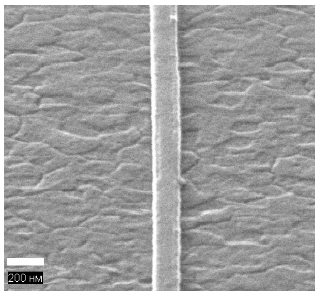
Рис.5. РЭМ фотография вытравленного рельефа активной области с удаленной резистивной маской по режиму с промежуточным охлаждением ( RF = 125 W, ICP = 50 W)
